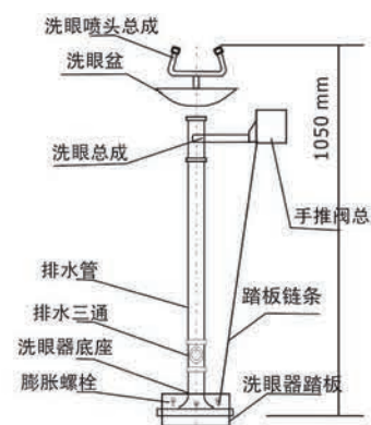
◎BTL61-A 立式紧急洗眼器 304+ABS防腐涂层（可选碳钢） BTL61-A Vertical emergency eye washer 304 +ABS corrosionproof coating (carbon steel is optional)
